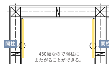
〈俯瞰図〉スリム側板
