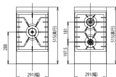
【平面図】
