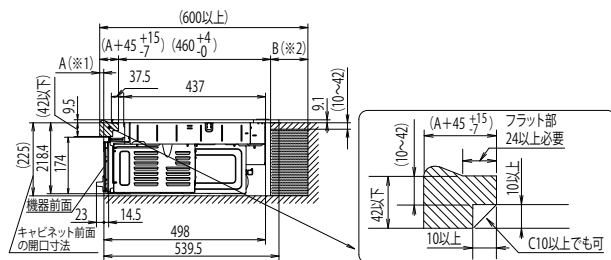
【側面図】
