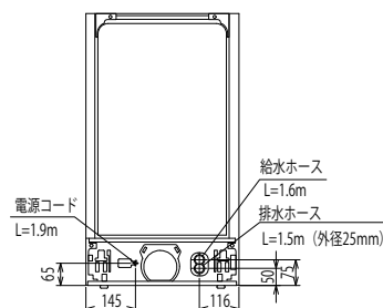
【背面図】
