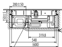
【背面図】
