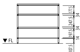
正面図 (壁際)
