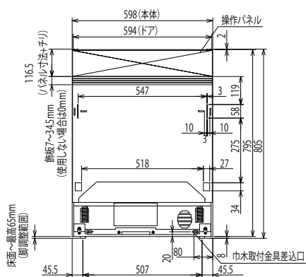
【正面図】
