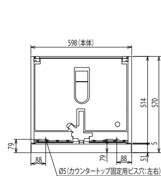
【平面图】
