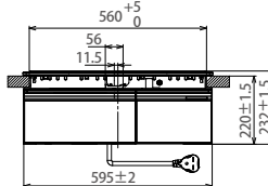
【正面図】
