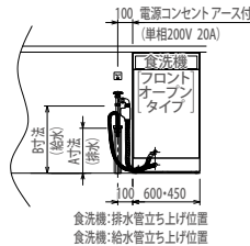
〈縦配管〉配管位置例図
