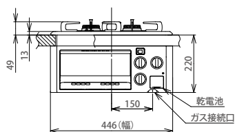
【正面図】
