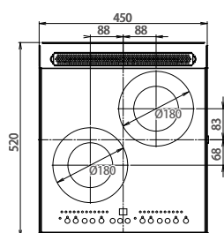
【平面図】
