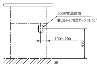
電源コンセント位置図
