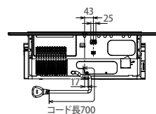
【背面図】
