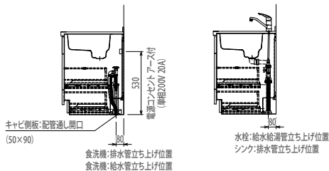
〈横配管〉配管位置例図
