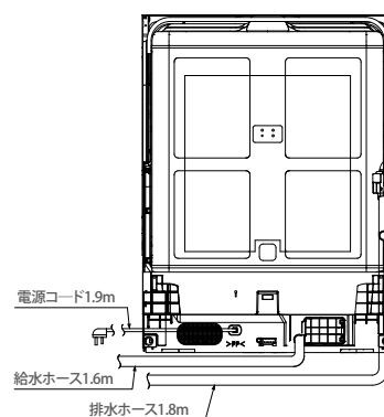
【背面図】
