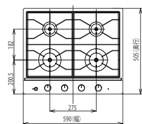
【平面図】
