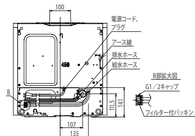
【背面図】
