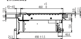
【側面図】
