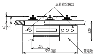
【正面図】
