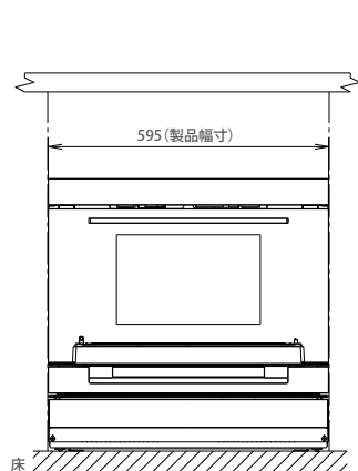
【正面図】
