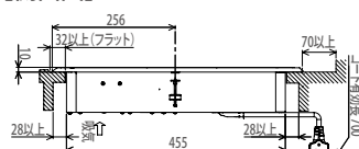
【側面図】
