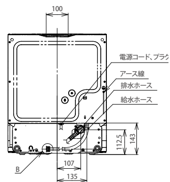
【背面図】
