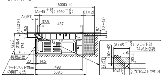
【側面図】
