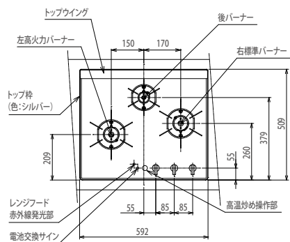
【平面図】
