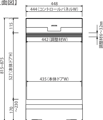
【正面図】
