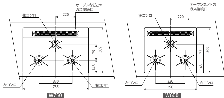
【平面図】
