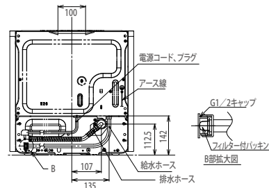
【背面図】
