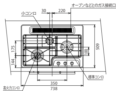
【平面図】
