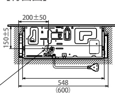
【背面図】
