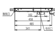
【側面図】
