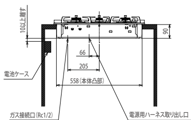
【正面図】
