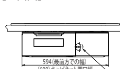
【正面図】
