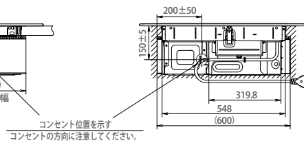
【背面図】
