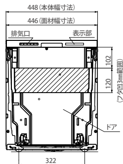
【正面図】
