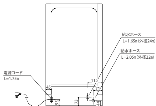
【背面図】
