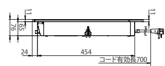
【側面図】
