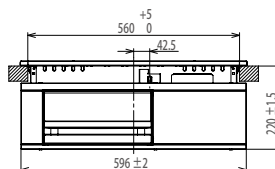
【正面図】
