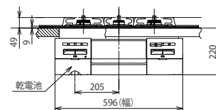
【正面図】
