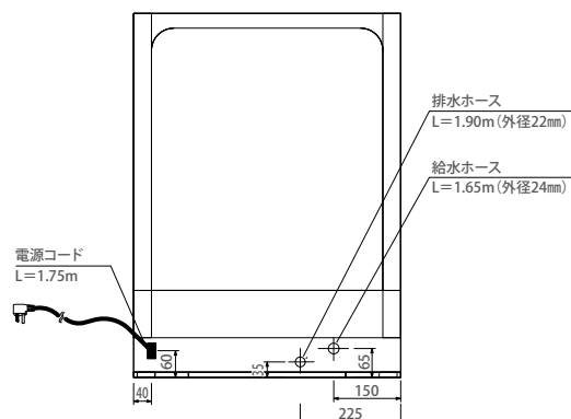
【背面図】
