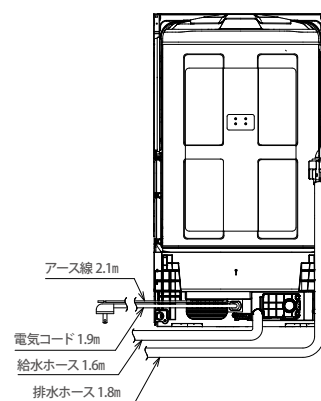
【背面図】
