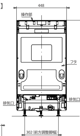
【背面図】
