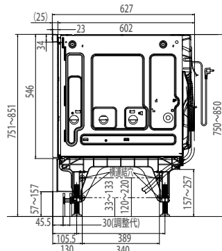
【側面図】
