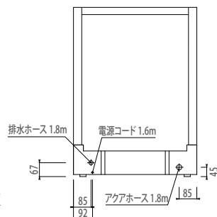
【背面図】
