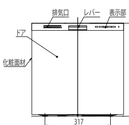
【正面図】
