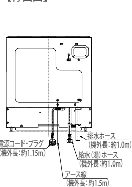
【背面図】
