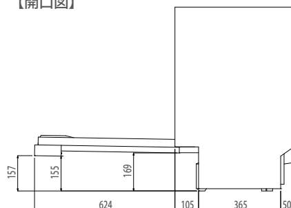
【開口図】
