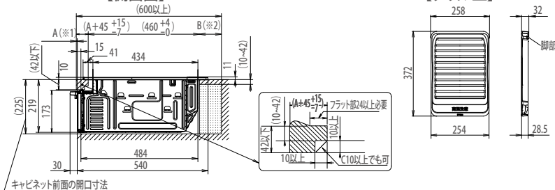
【側面図】
