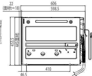
【側面図】
