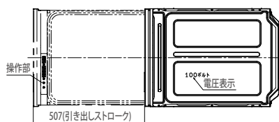
【平面図】
