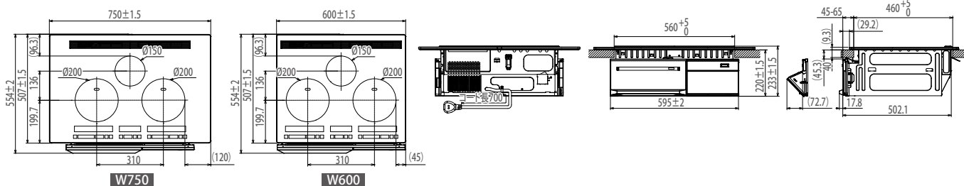
【平面図】
