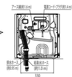
【背面図】
