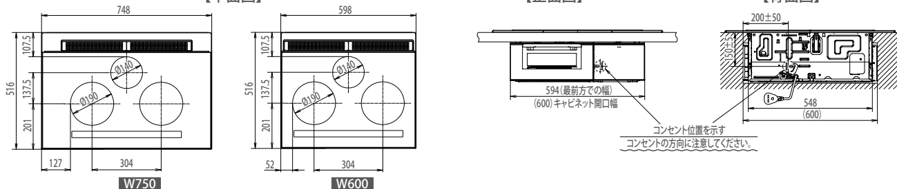
【側面図】
