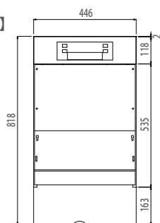
【正面図】
