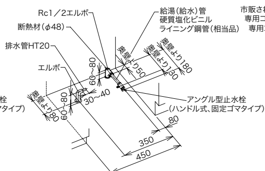
床立ち上げの配管例
