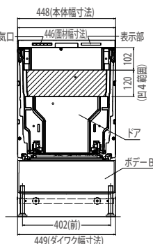
【正面図】
