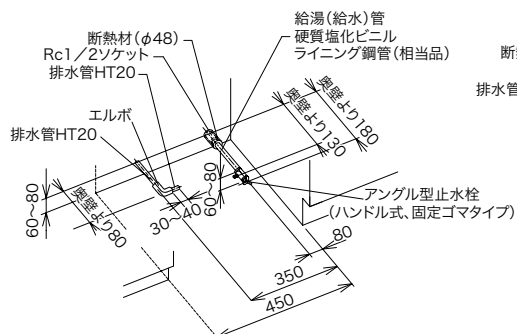
壁出しの配管例
