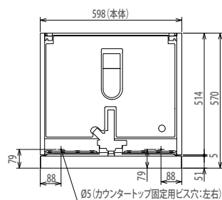
【側面図】
