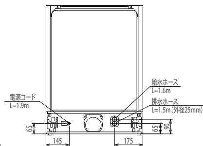
【背面図】
