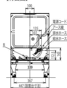
【背面図】
