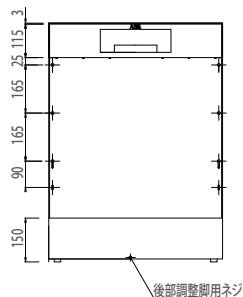
【正面図】
