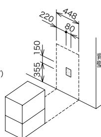
コンセントの取り付け位置 (キッチン高さ850mmの場合)
