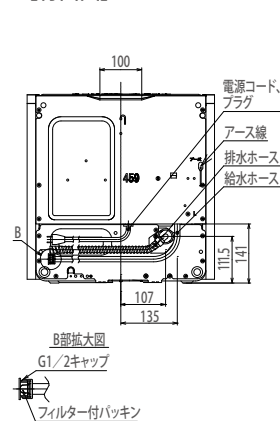
【背面図】
