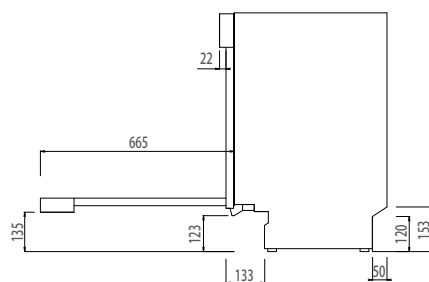
【右側面図】
