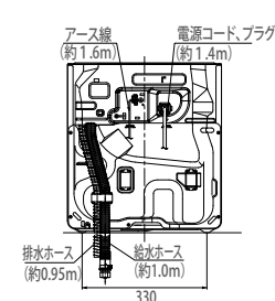
【背面図】
