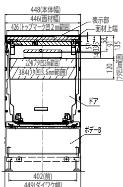
【正面図】
