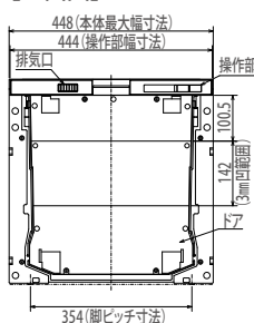
【正面図】
