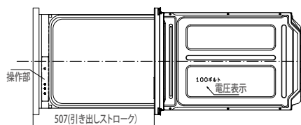
【平面図】
