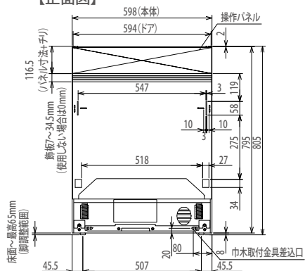
【正面図】
