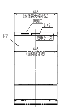
【正面図】
