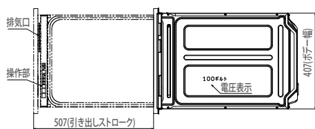
【平面図】
