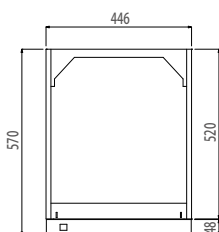
【開口図】
