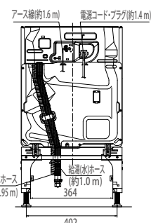
【背面図】
