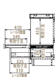
【引出し寸法図】
