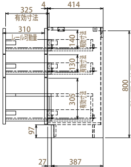
【引出し寸法図 D=450】
