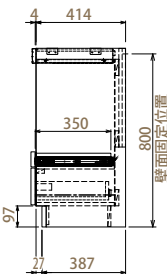
【側面図】
