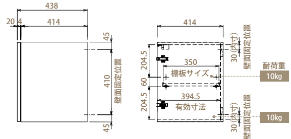
【キャビネット内図 片開き (W:450)】
