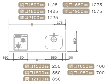
ワークトップ俯瞰図
