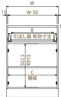
【キャビネット内図】
