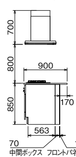
■レンジフード側面図
