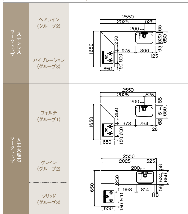
サイドパネルなし納まり(W2550)
