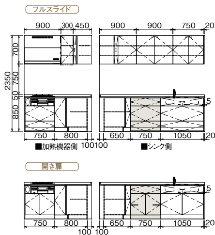
サイドパネルあり納まり(W2575)
