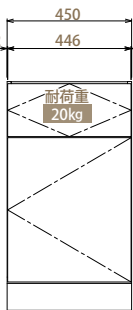
【正面図 片開き(W:450)】
