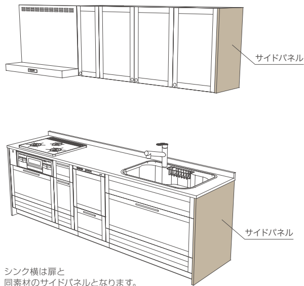
片側オープンの場合の納まり（サイドパネルあり）
