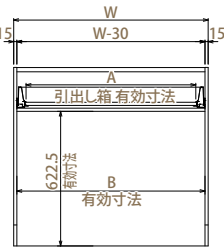
【キャビネット内図】
