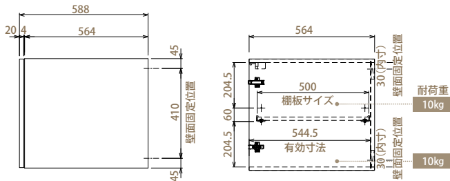
【キャビネット内図 両開き (W:900/750/600)】
