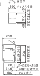
キャビネット側断面図
