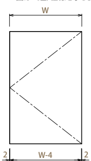
【正面図 片開き】
