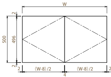
【側面図 D=600】
