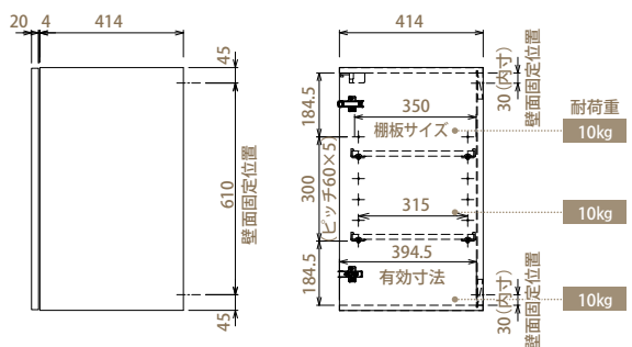
【側面図 D=450】
