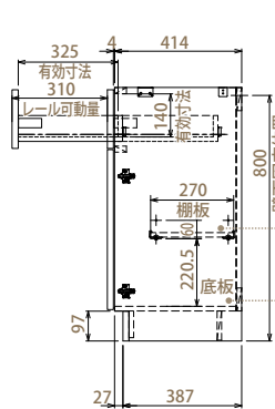
【引出し寸法図 D=450】
