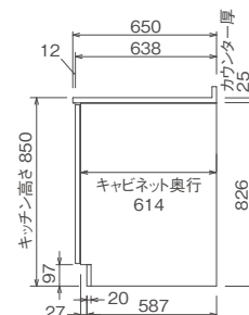
〈キャビネット断面図〉
