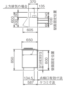
レンジフード側断面図
