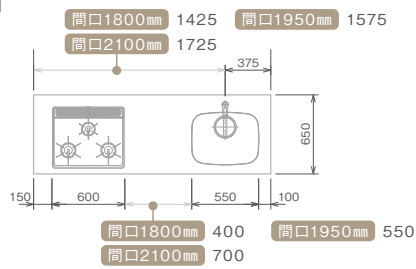
ワークトップ俯瞰図
