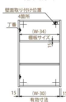
【キャビネット内図 片開き (W:450)】
