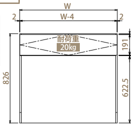
【正面図】
