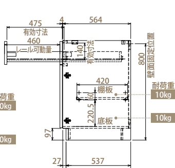
【引出し寸法図 D=600】
