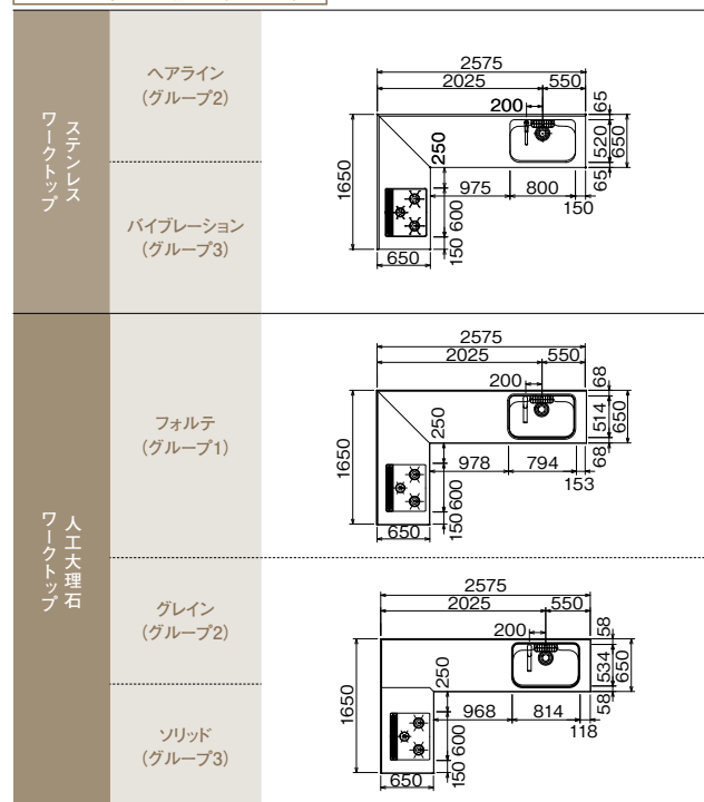
サイドパネルあり納まり(W2575)
