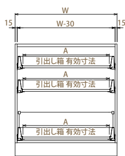
【キャビネット内図】
