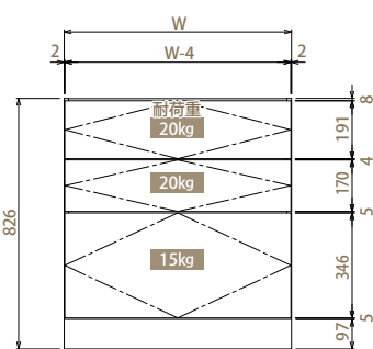
【正面図】
