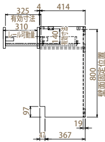
【引出し寸法図 D=450】
