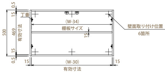
【キャビネット内図 両開き (W:900/750/600)】
