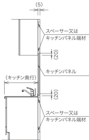
＜キッチンパネル先付け納まり＞
