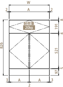
【正面図 両開き(W:600/750/900)】
