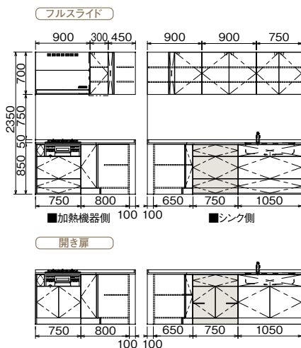
サイドパネルなし納まり(W2550)
