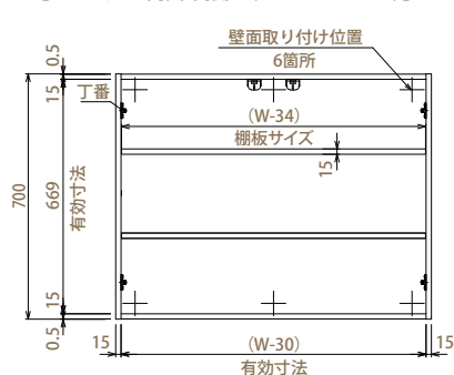
【キャビネット内図 両開き (W:900/750/600)】
