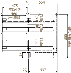
【引出し寸法図 D=600】
