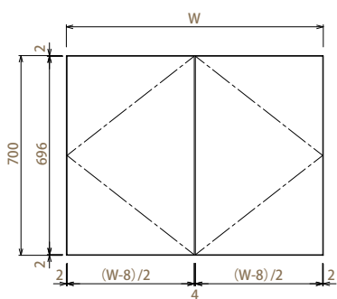
【正面図 両開き】
