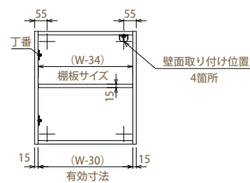
【キャビネット内図 片開き (W:450)】
