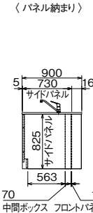
■キャビネット側面図
