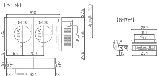
ガス機器-寸法図
