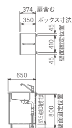
■キャビネット側断面図
