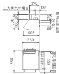
■キャビネット側断面図
