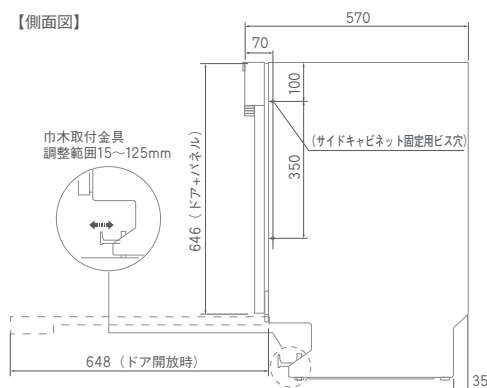
【側面図】
