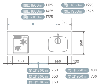
ワークトップ俯瞰図
