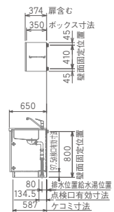
キャビネット側断面図
