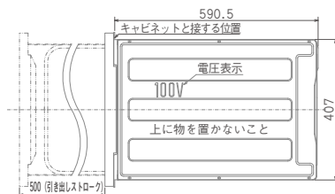
【上面図】
