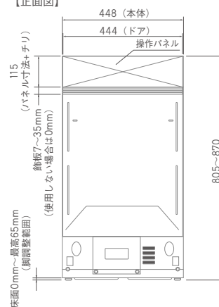
【正面図】
