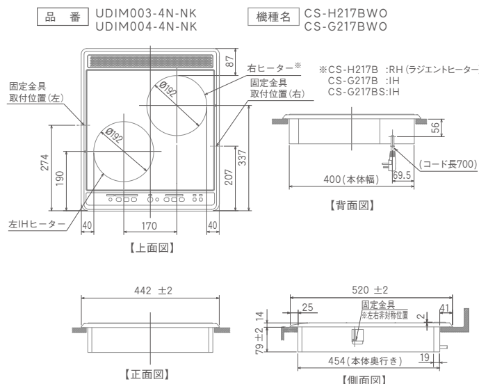
IH機器-寸法図
