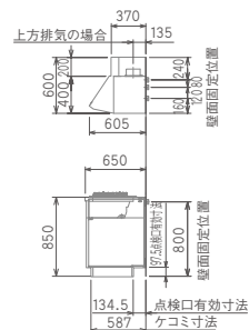
キャビネット側断面図
