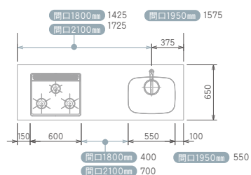
ワークトップ俯瞰図
