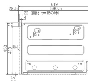
【側面図】
