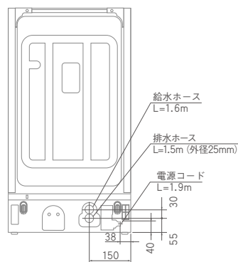
〈横配管〉各シンク別配管位置例図
